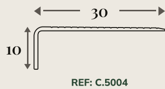
Cantoneira 30x10
